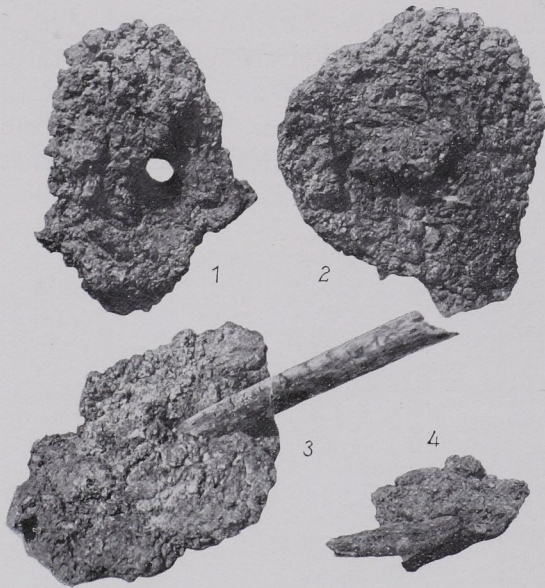
Fig. 39 Strengflüssige Rohschlackenklöße.
