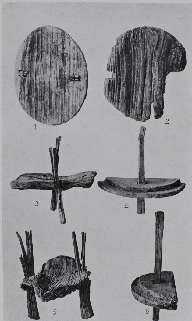
Fig. 11 Konstruktive Details der Wasserkübel. \frac{1}{5-3} n. Gr.
