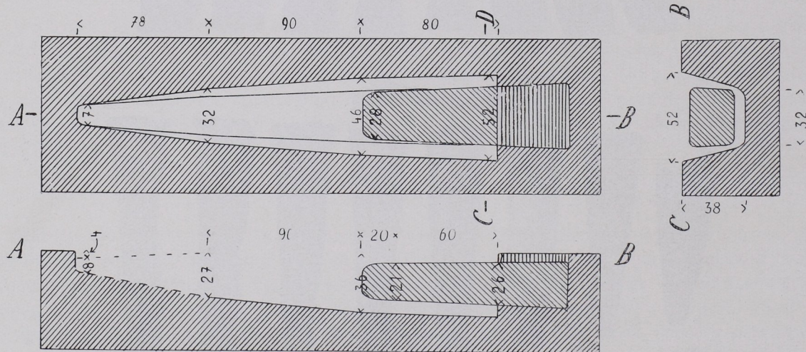
Fig. 30 Rekonstruktion der Gußform des Pickels Fig. 29, 4 (Ansicht von oben, Längs- und Querschnitt). Maße in Millimetern.
