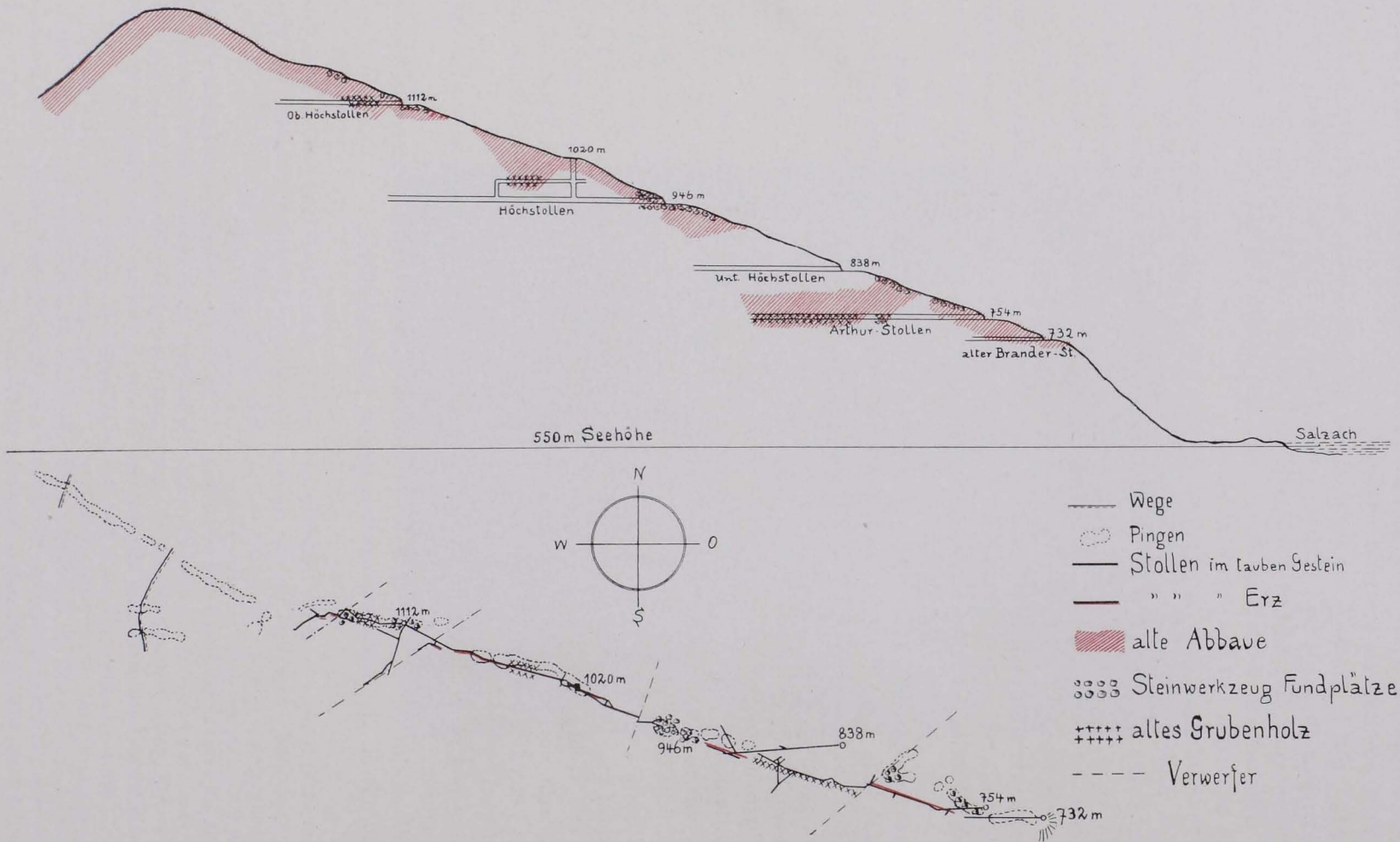
Fig. 14 Grundriß und Aufriß der Stollen, Pingen und alten Abbaue am Brandergange (Einödtberg).
