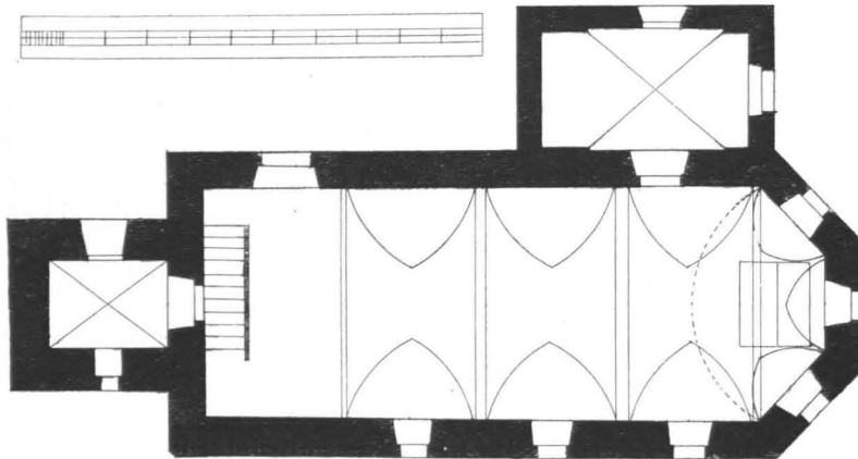
Fig. 181 Waldprechting, Filialkirche, Grundriß 1 : 200 (S. 184)
