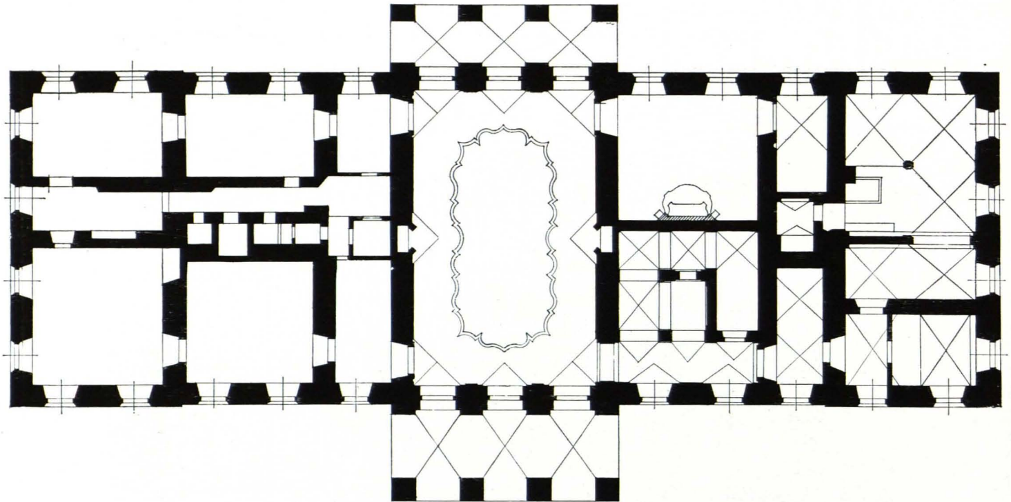
Fig. 274 Leopoldskron. Grundriß im Erdgeschoß 1 : 300 (S. 308)
