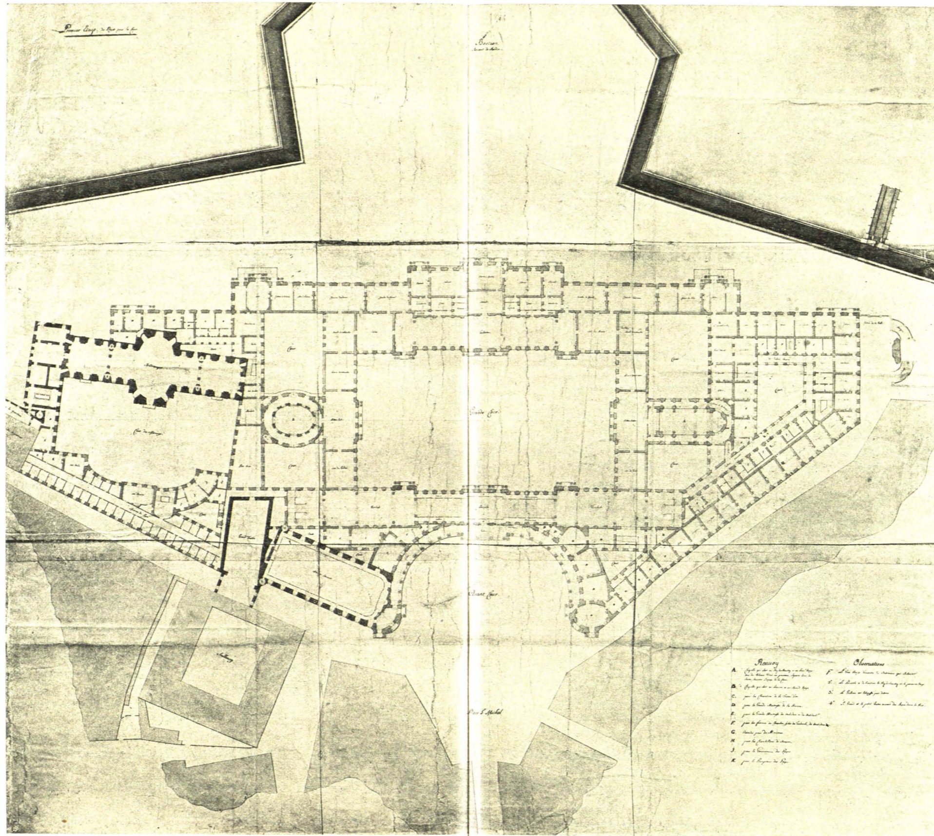
Abb. 269 Grundriß des ersten Obergeschosses zu dem Entwurfe auf Abb. 266, k. k. Hofbibliothek A. Kapelle im Parterre und 1. Stock (vgl. Abb. 283) B. Kapelle im 1. und 2. Stock (vgl. Abb. 284)
