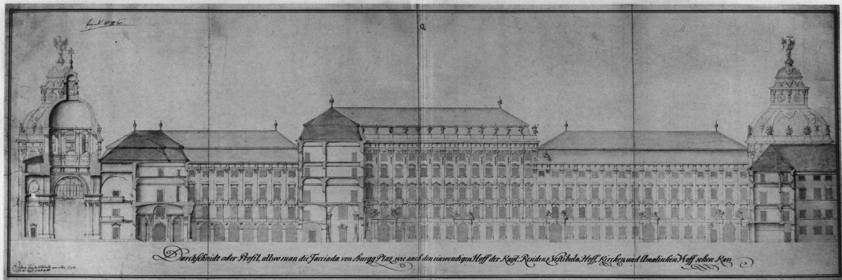
Abb. 210 Durchschnitt durch die von Joh. Luk. v. Hildebrandt geplanten Burghöfe in der Richtung von Südost nach Nordwest, signiert und datiert 1725, in der k. k. Hofbibliothek
