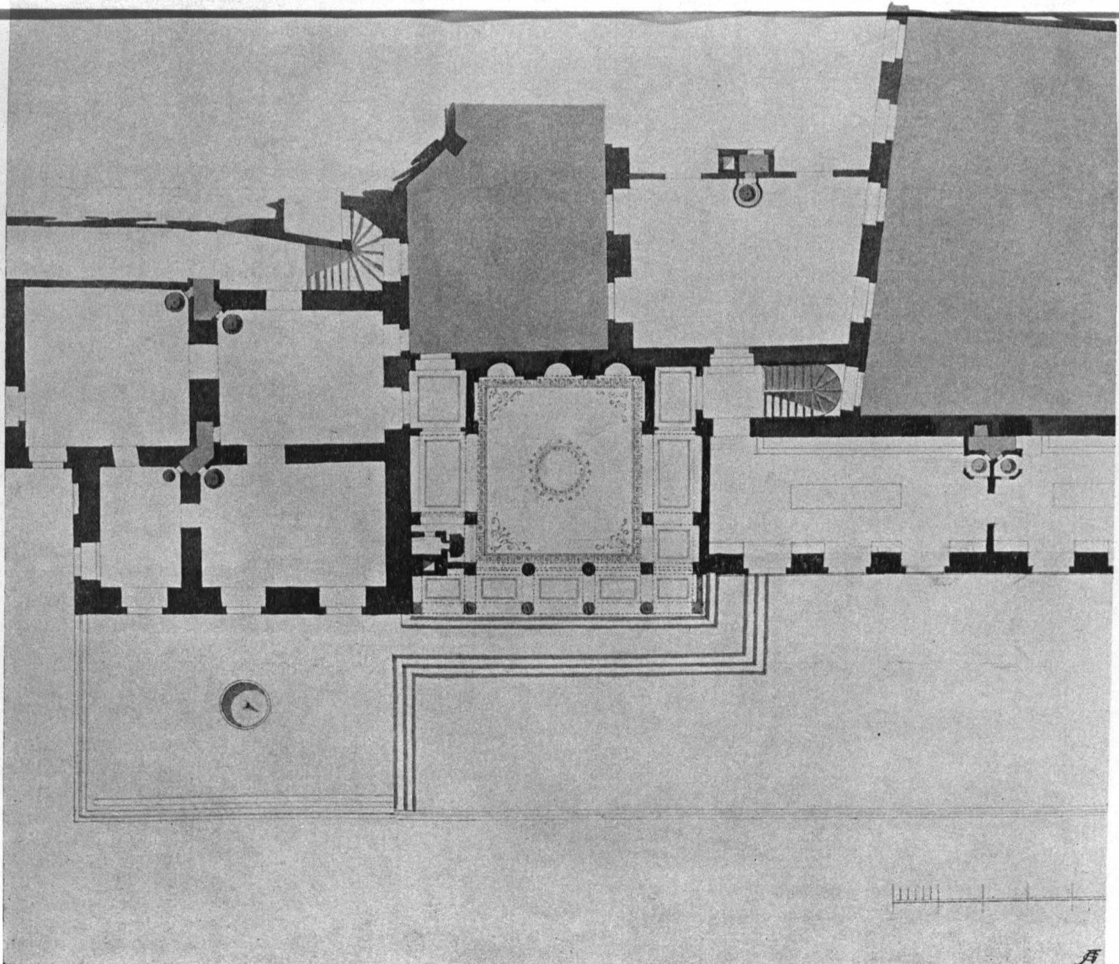
Abb. 66, 67 Ausschnitte aus einem Entwurfe zur Umgestaltung der Gartenterrasse über dem Naturalienkabinette aus der Zeit des Kaisers Franz I. (II.)
