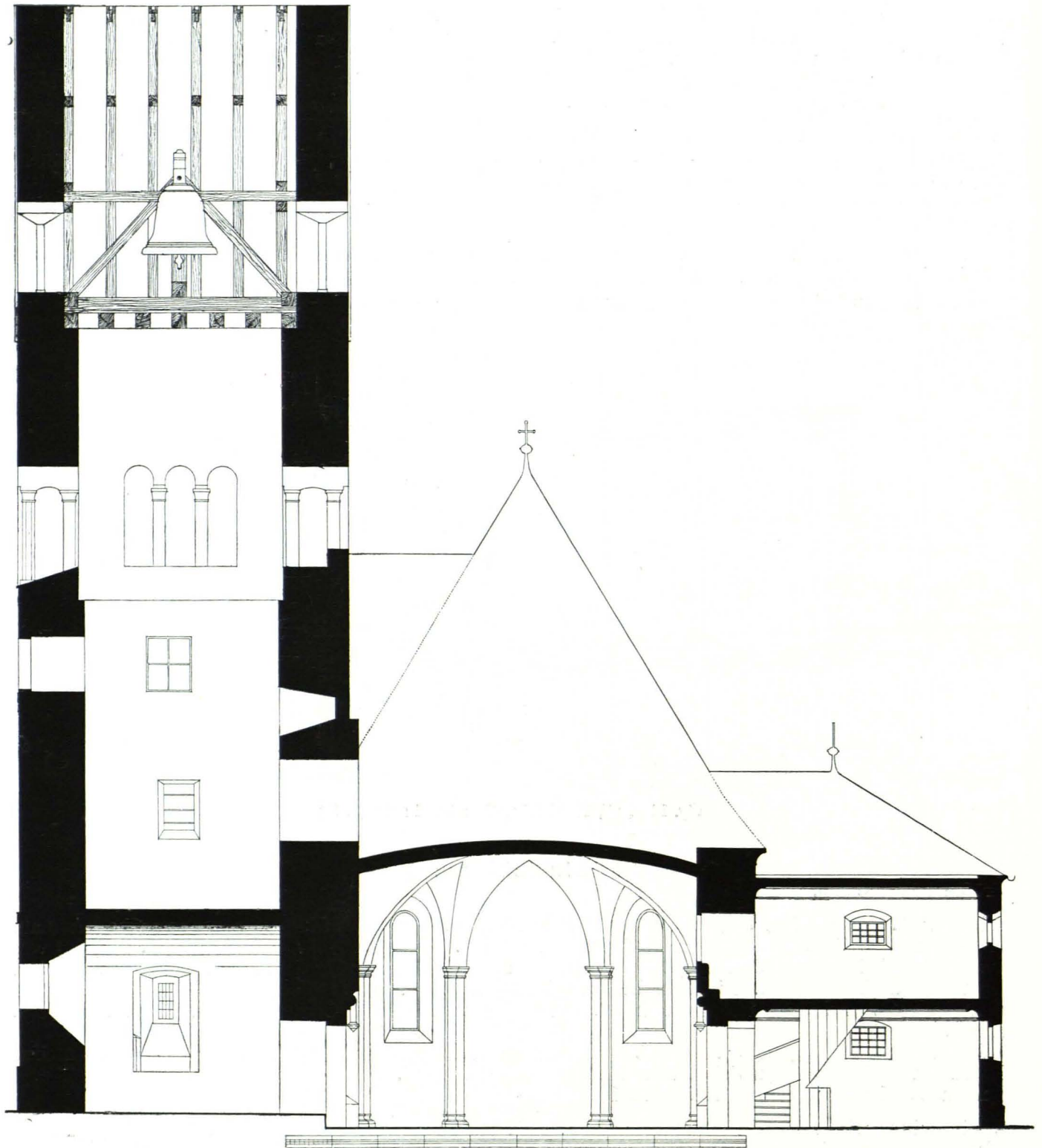
Fig. 15 Anif, Pfarrkirche, Querschnitt 1 : 250 (S. 14)
