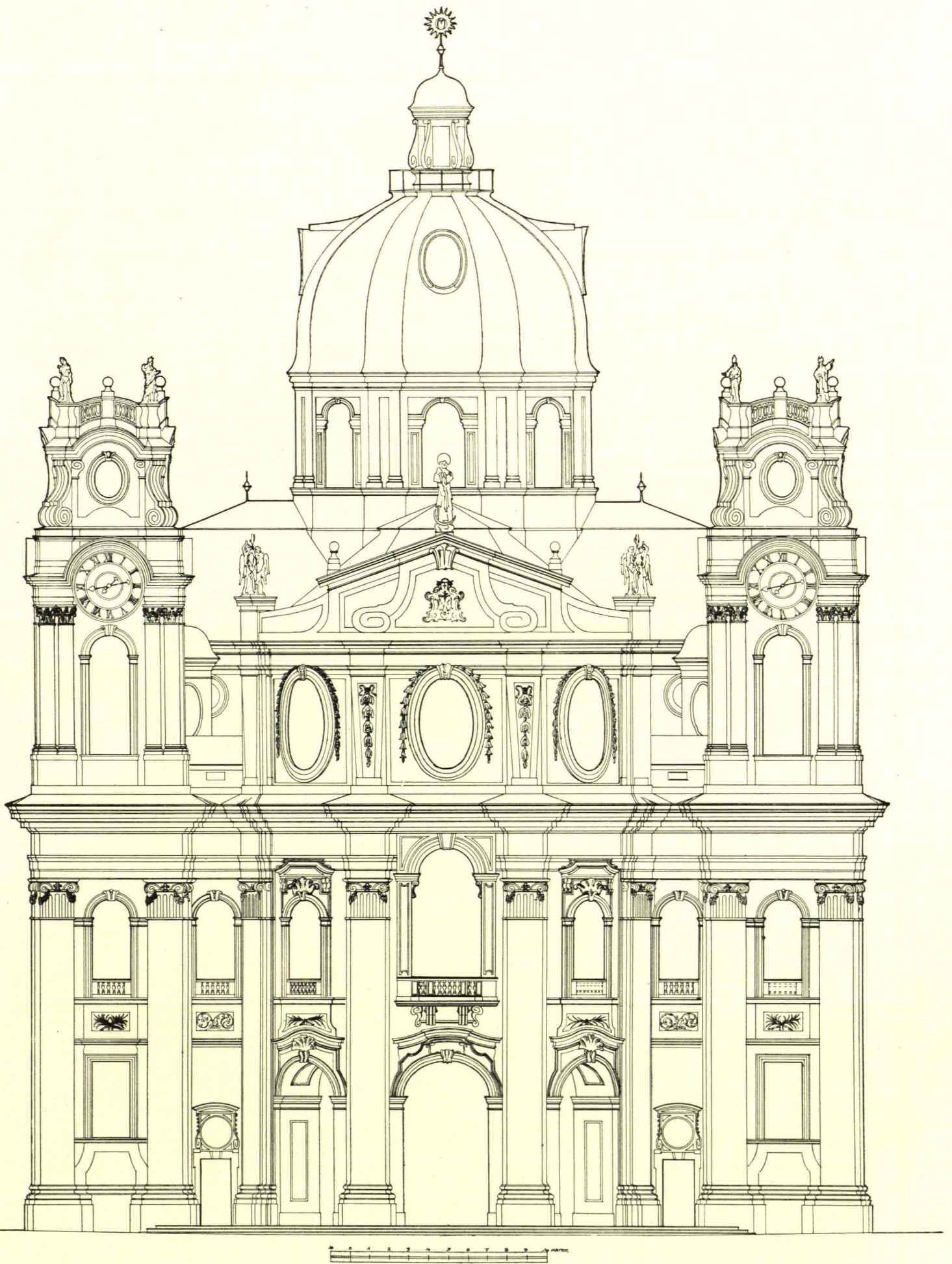
TAFEL XXXIV KOLLEGIENKIRCHE, FASSADE 1 : 250 (S. 242)
