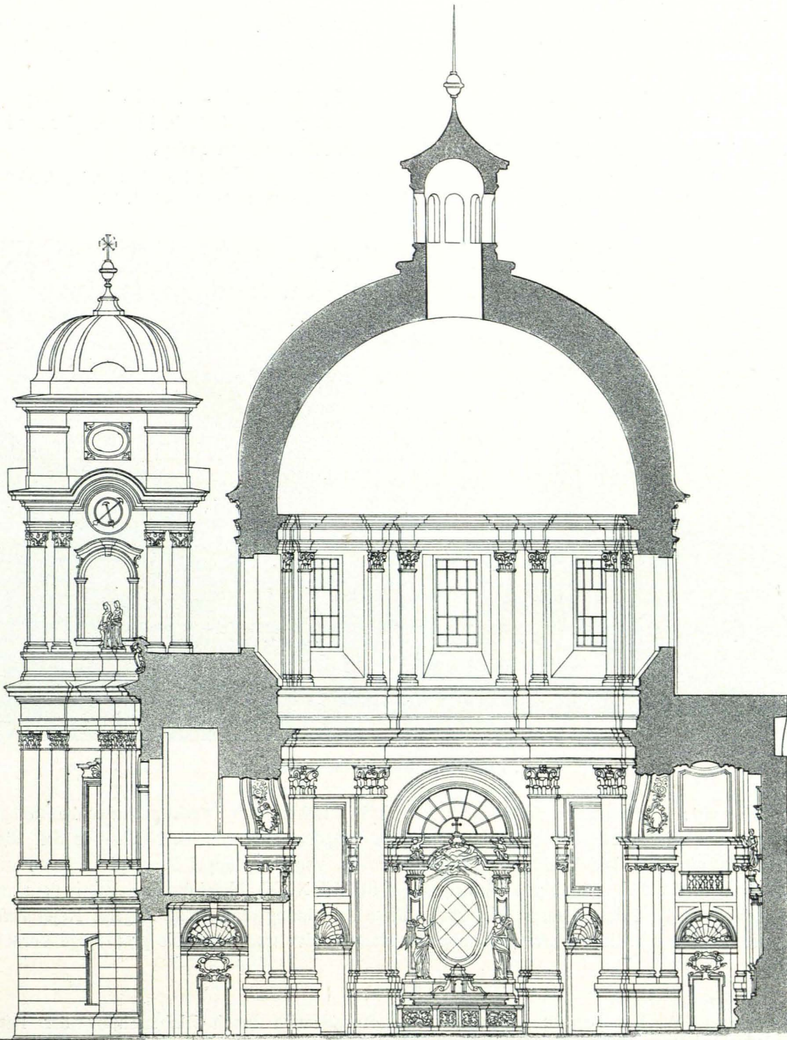
Fig. 191 Dreifaltigkeitskirche, Längsschnitt 1 : 200 (S. 164)
