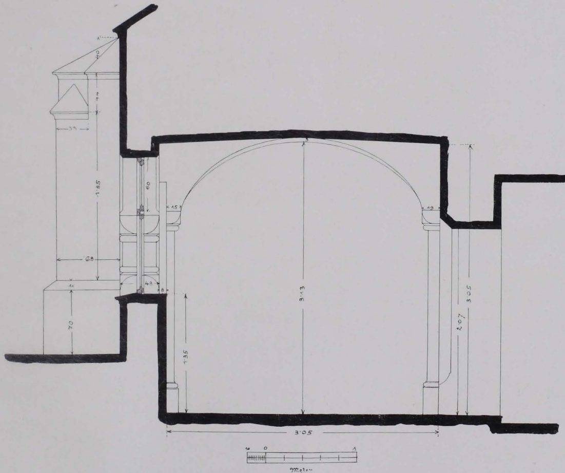
Fig. 84 Kreuzgang, Querschnitt durch ein Gewölbejoch 1:40 (S. 64)
