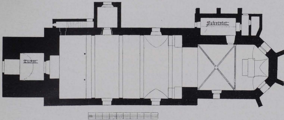
Fig. 1 Dobersberg, Pfarrkirche, Grundriß 1 : 300 (S. 2)
