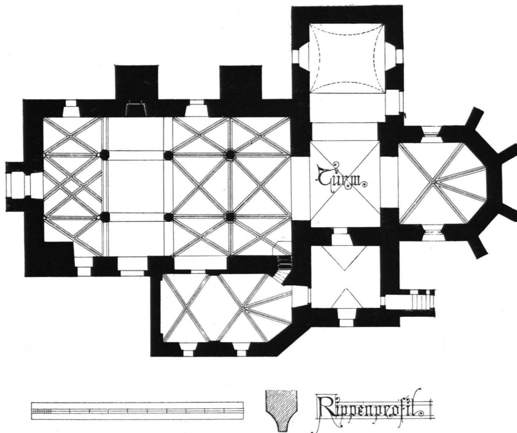
Fig. 345 Rieggers, Pfarrkirche, Grundriß 1 : 200 (S. 373)
