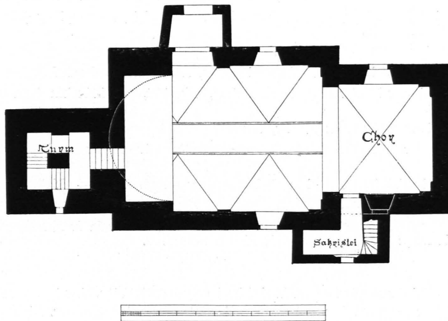
Fig. 336 Nieder-Nondorf, Pfarrkirche, Grundriß 1 : 200 (S. 358)
