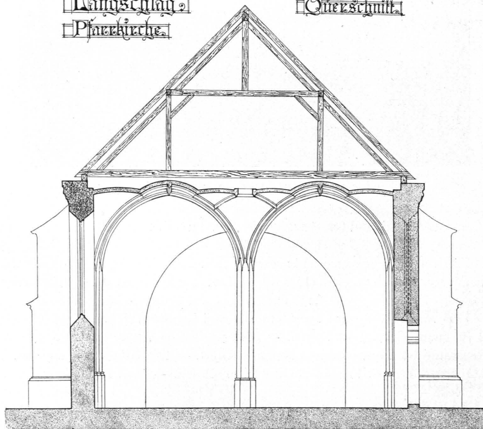
Fig. 217 Langschlag, Pfarrkirche, Querschnitt durch das Langhaus, 1 : 125 (S. 248)
