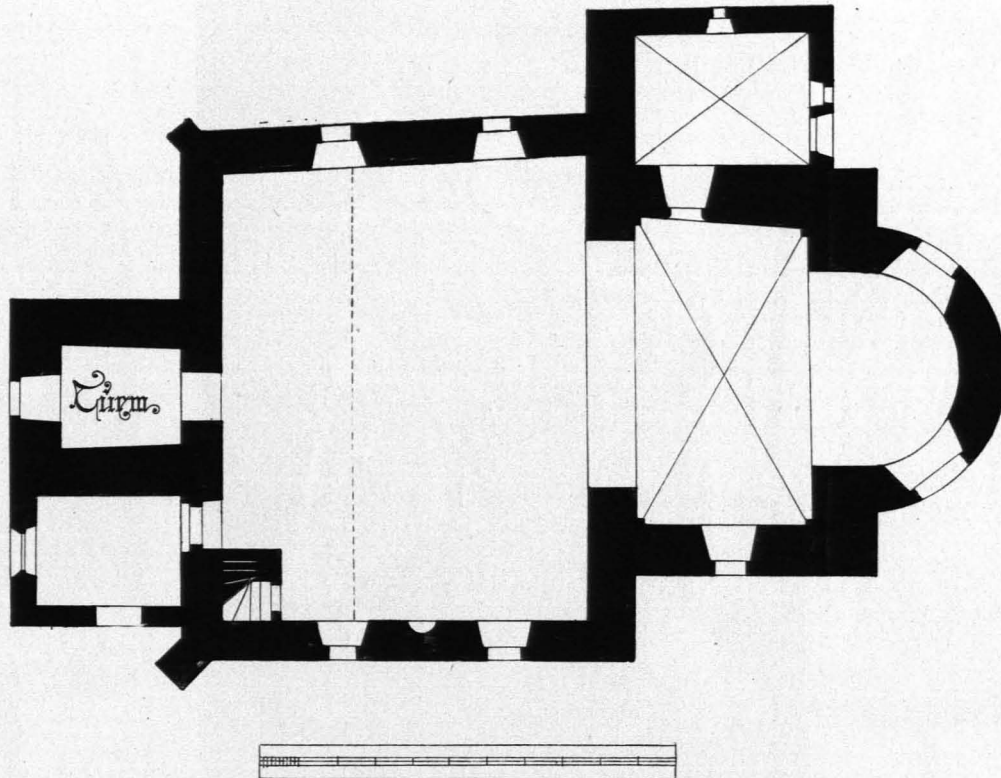
Fig. 381 Waldhausen, Pfarrkirche, Grundriß 1 : 200 (S. 415)
