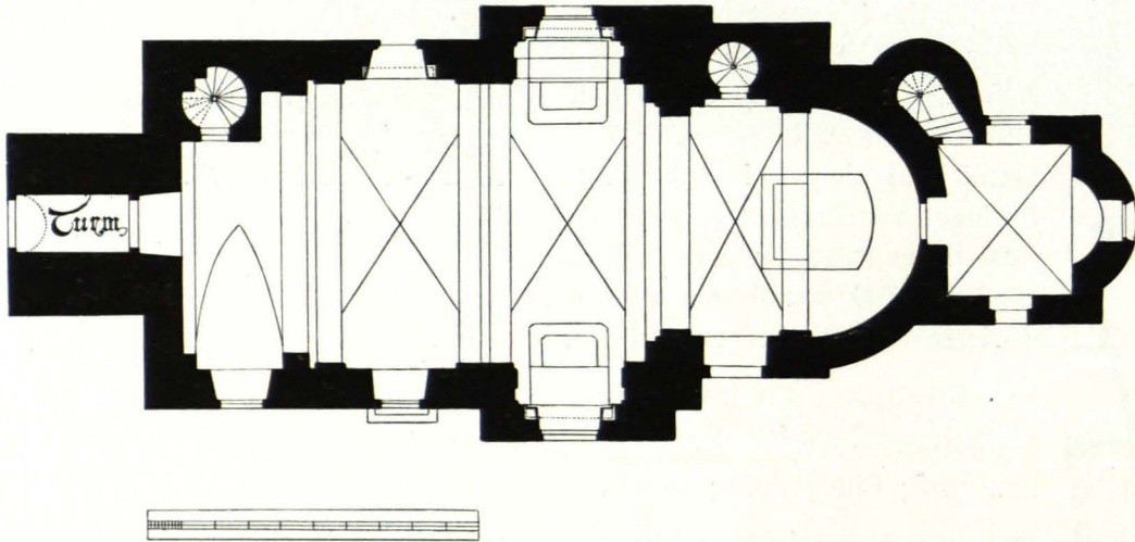
Fig. 296 Pisching, Pfarrkirche, Grundriß 1 : 250 (S. 249)
