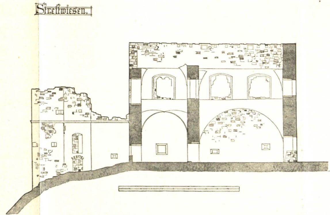
Fig. 122 Streitwiesen, Ruine, Querschnitt (S. 116)
