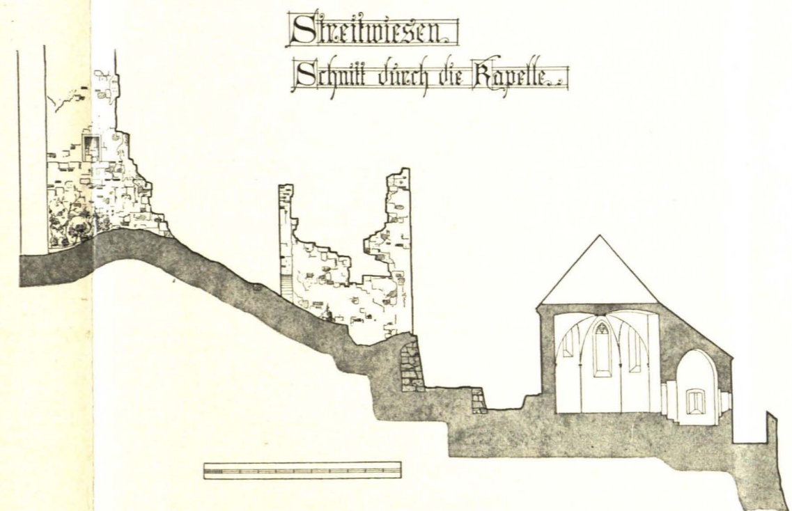
Fig. 123 Streitwiesen, Ruine, Schnitt durch die Kapelle (S. 116)
