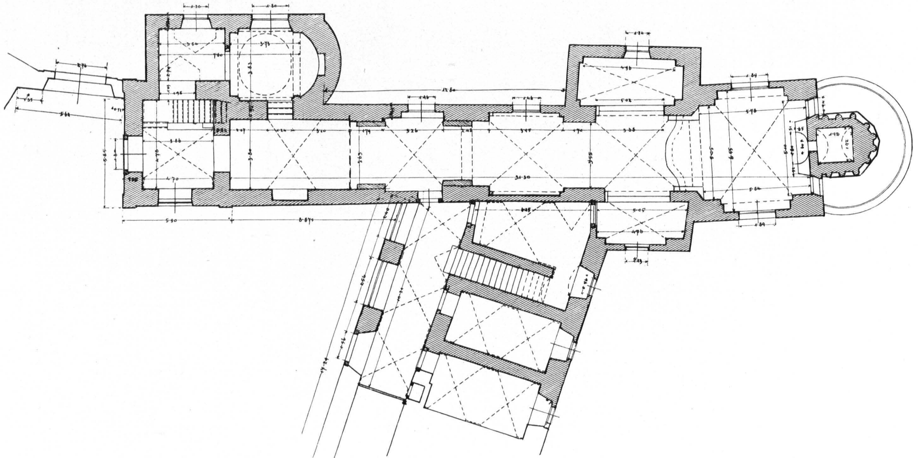
Fig. 441 Schönbüchel, Grundriß der Kirche (S. 423)
