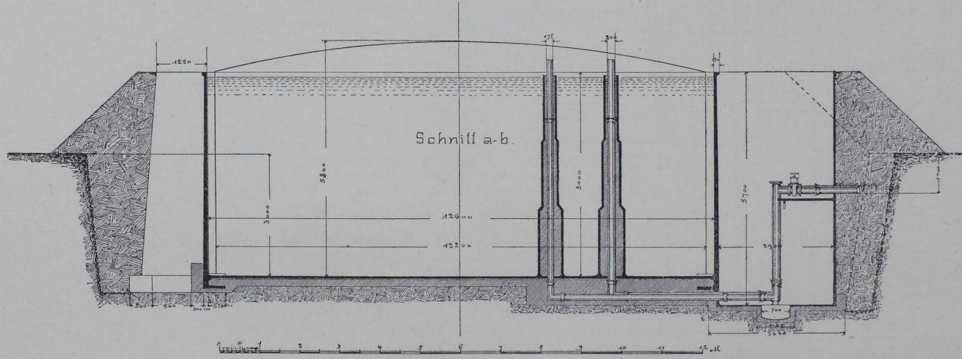
Durchschnitt mit Ansicht einer Pfeilervorlage.
