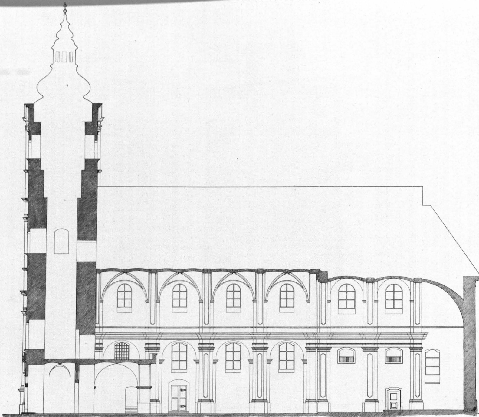
Fig. 145 Loosdorf, Pfarrkirche, Längsschnitt (S. 117)
