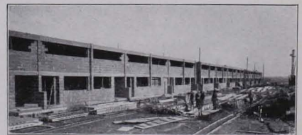
Abb. 111 SIEDLUNG TÖRTEN, DESSAU 1926/27, im Bau (Beton)
