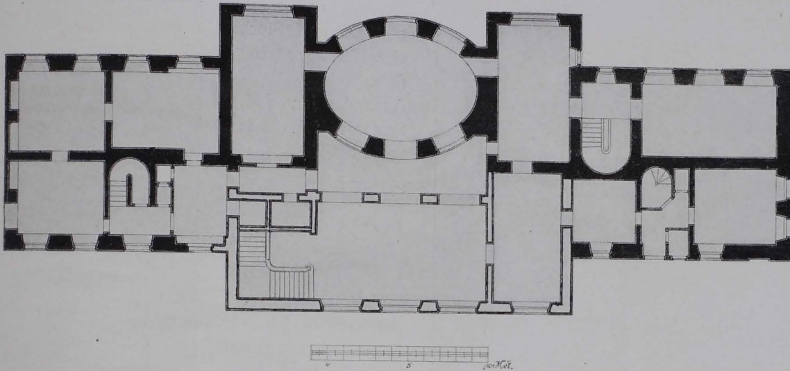
Fig. 272 Neuwaldegg, Schloß, Grundriß des Erdgeschosses (S. 250)
