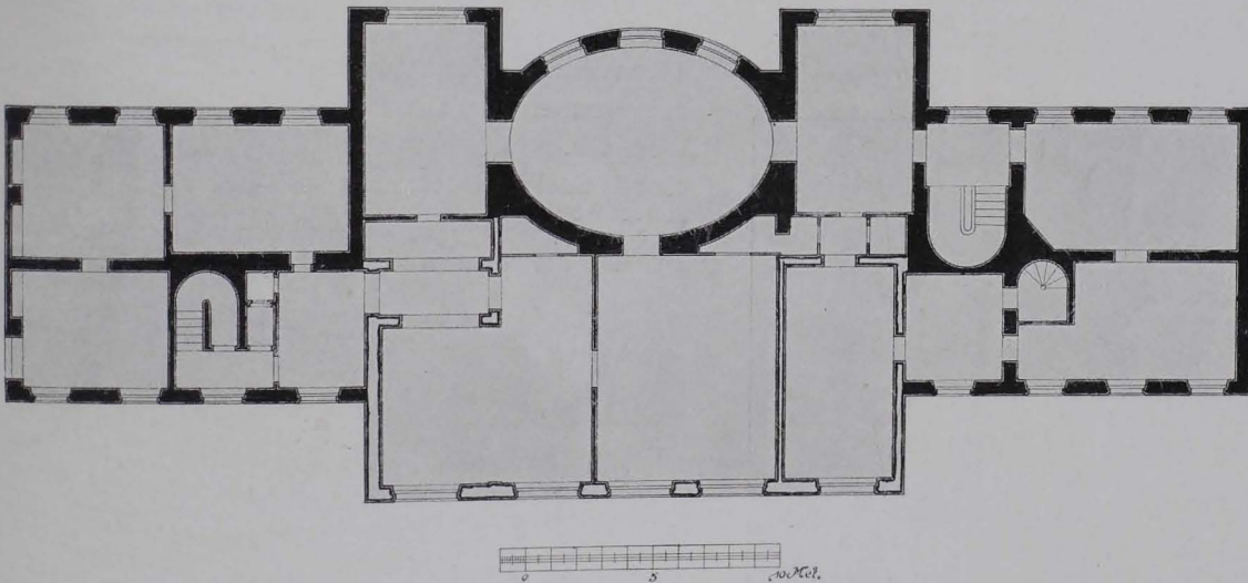
Fig. 273 Neuwaldegg, Schloß, Grundriß des ersten Stockes (S. 250)
