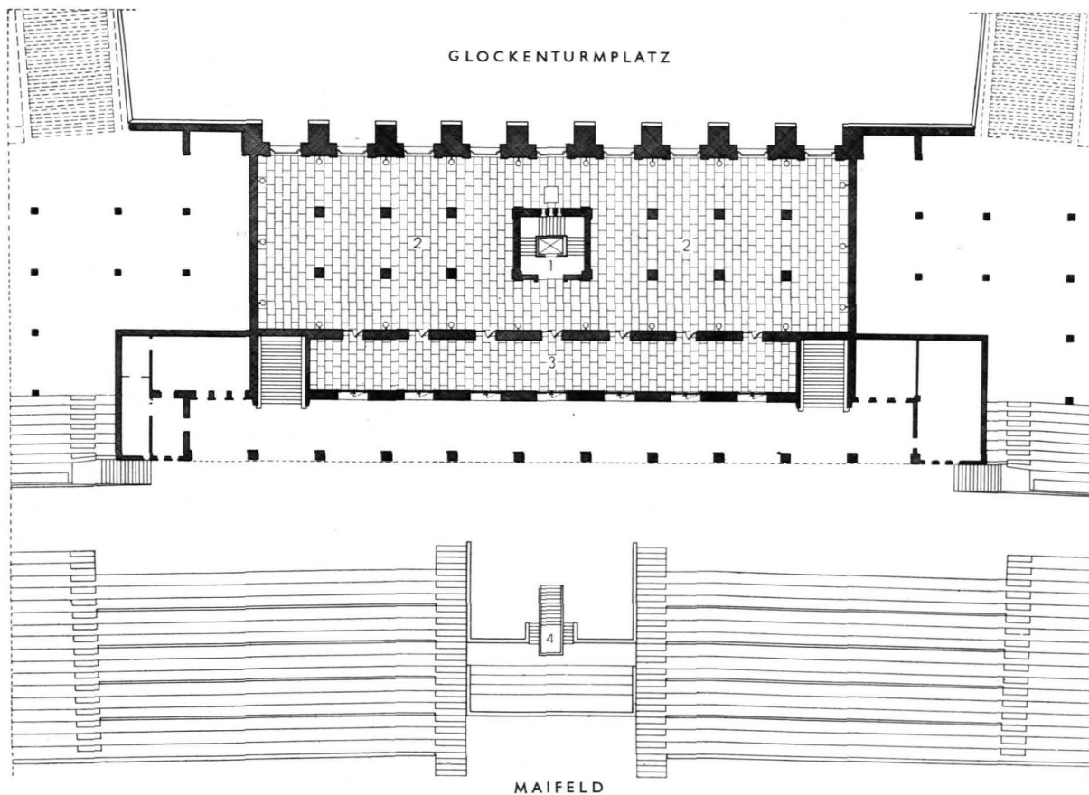
Abb. 12 Das Maifeld, Mitteltribüne. Grundriß
