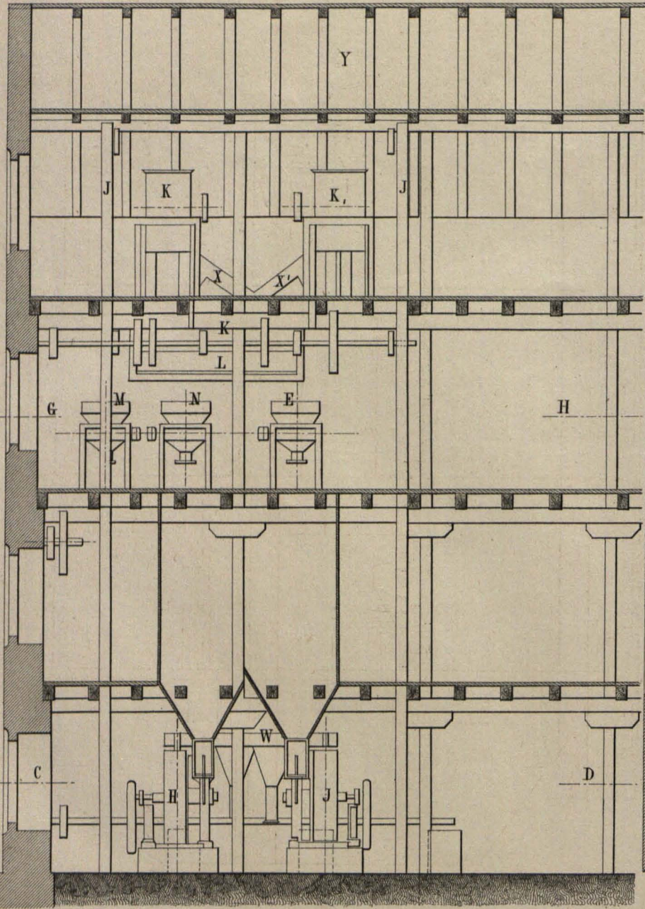
Längenschnitt A. B.
