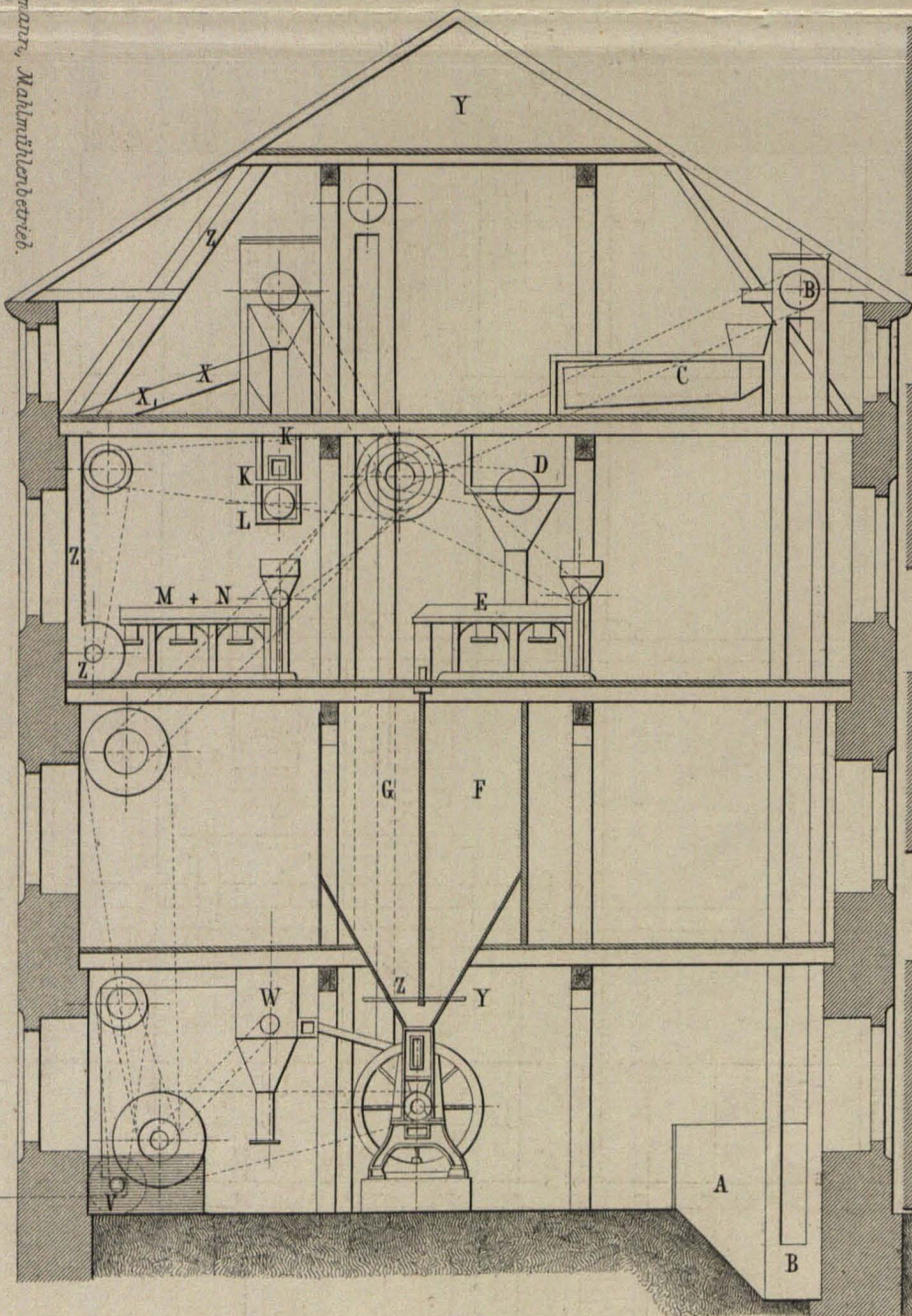
Querschnitt E. F.
