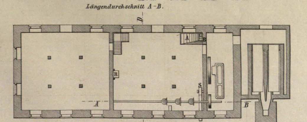
Fig. 5. Grundriss des Parterre.
