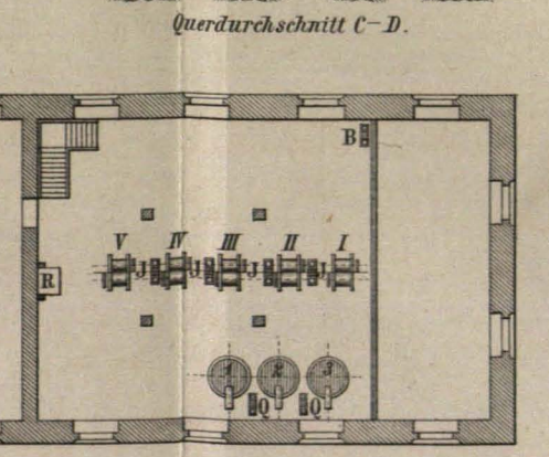
Fig. 4. Grundriss des Steinbodens.
