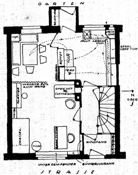
Abb. 55. Verbessertes Reihenhaus Erdgeschoß
