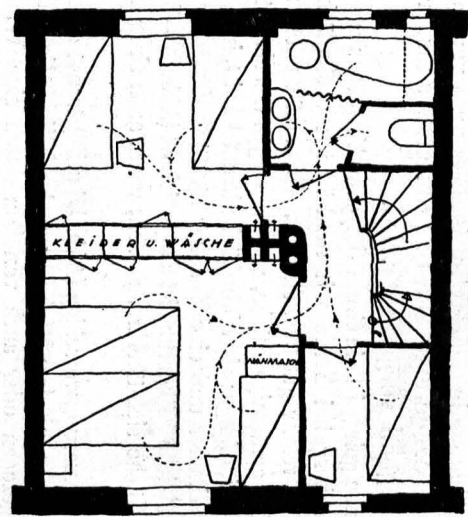
Abb. 56. Verbessertes Reihenhaus Obergeschoß
