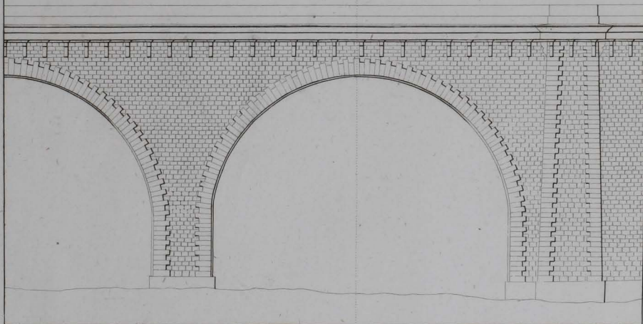
Aufsicht eines Theils der 5 mittelsten Bögen der Brückwasserleitung über das Thal bei Tourvoie. B
