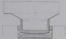
Durchschnitt und Grundriß des Zapfens und der Pfanne.
