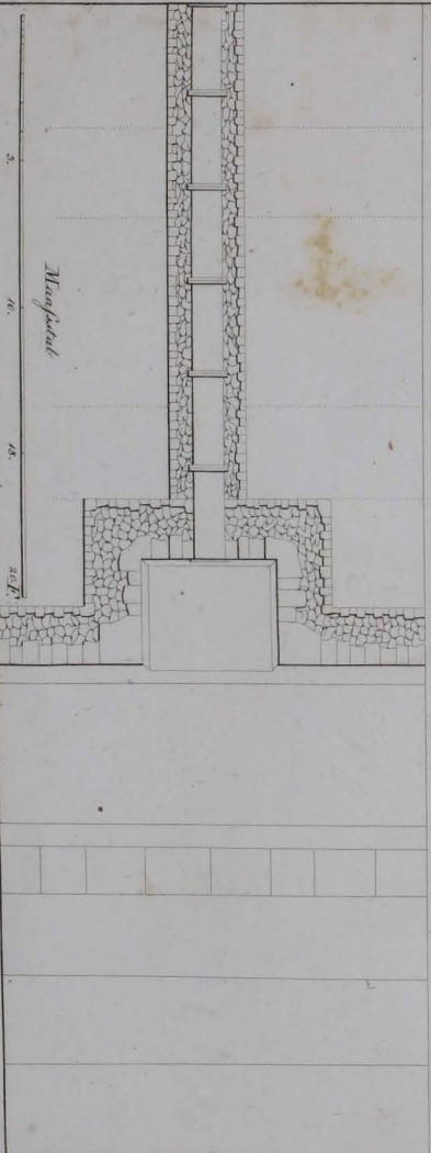
Grundriß und Durchschnitt der Ausmündung des Röhre, durch welche das Quellwasser von Bures her in den Yette Forni geleitet wird.
