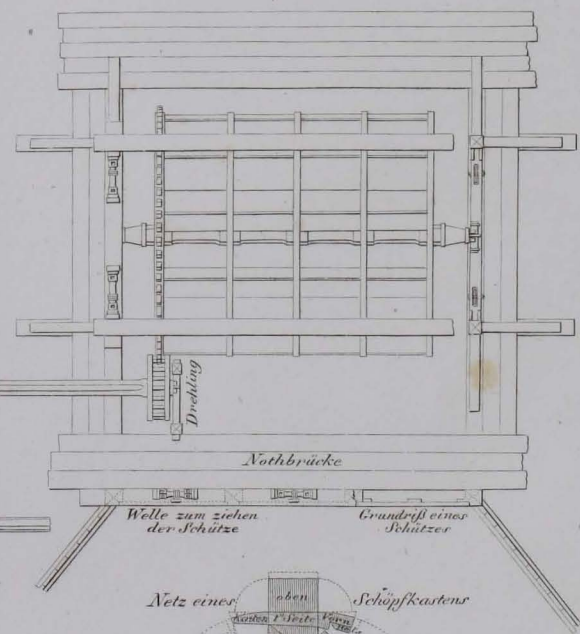
Grundriß eines Wasserrades mit Gerüste
