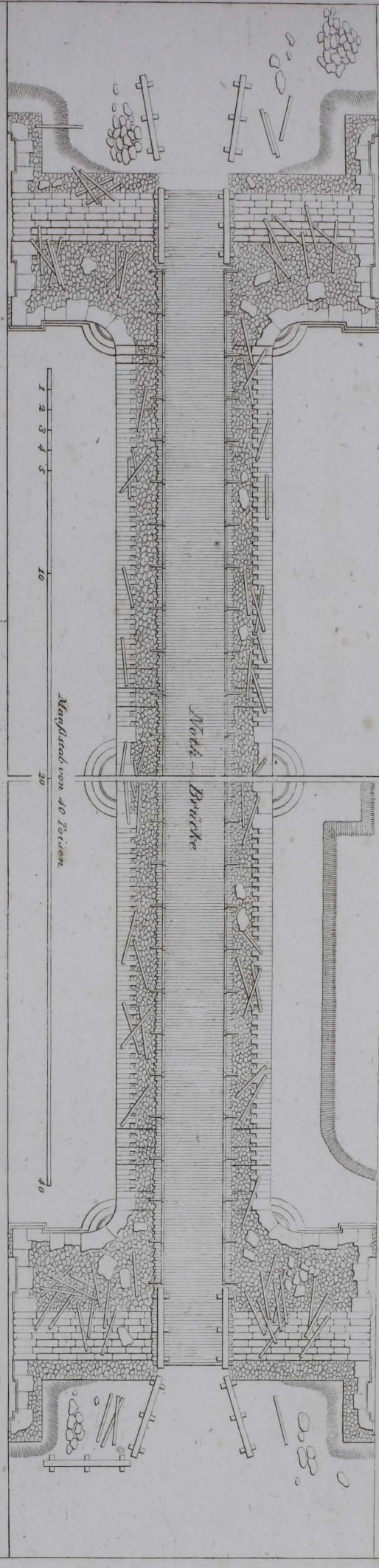
Grundriß Durchschnitt und Aufricht der Nothbrücke zum Abdämmen des Armes der Seine auf der Seite nach Paris zu.
