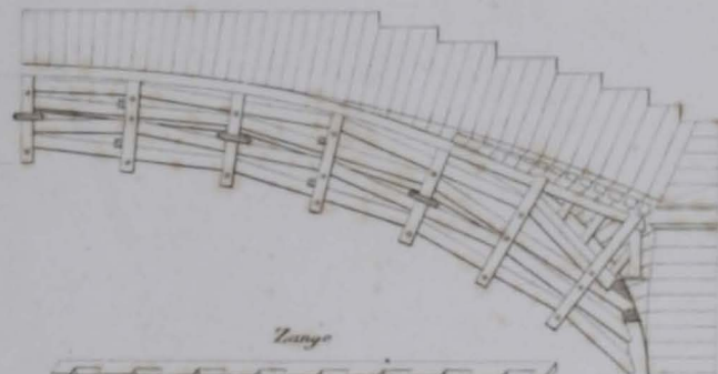
Grundriß der 8 Curven einer Lehrbögen
