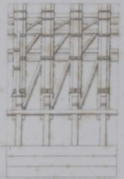
Verbindung der Hängebänder mit den Hängestützen
