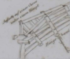
Teil einer Curve unter einem Haupt von innen
