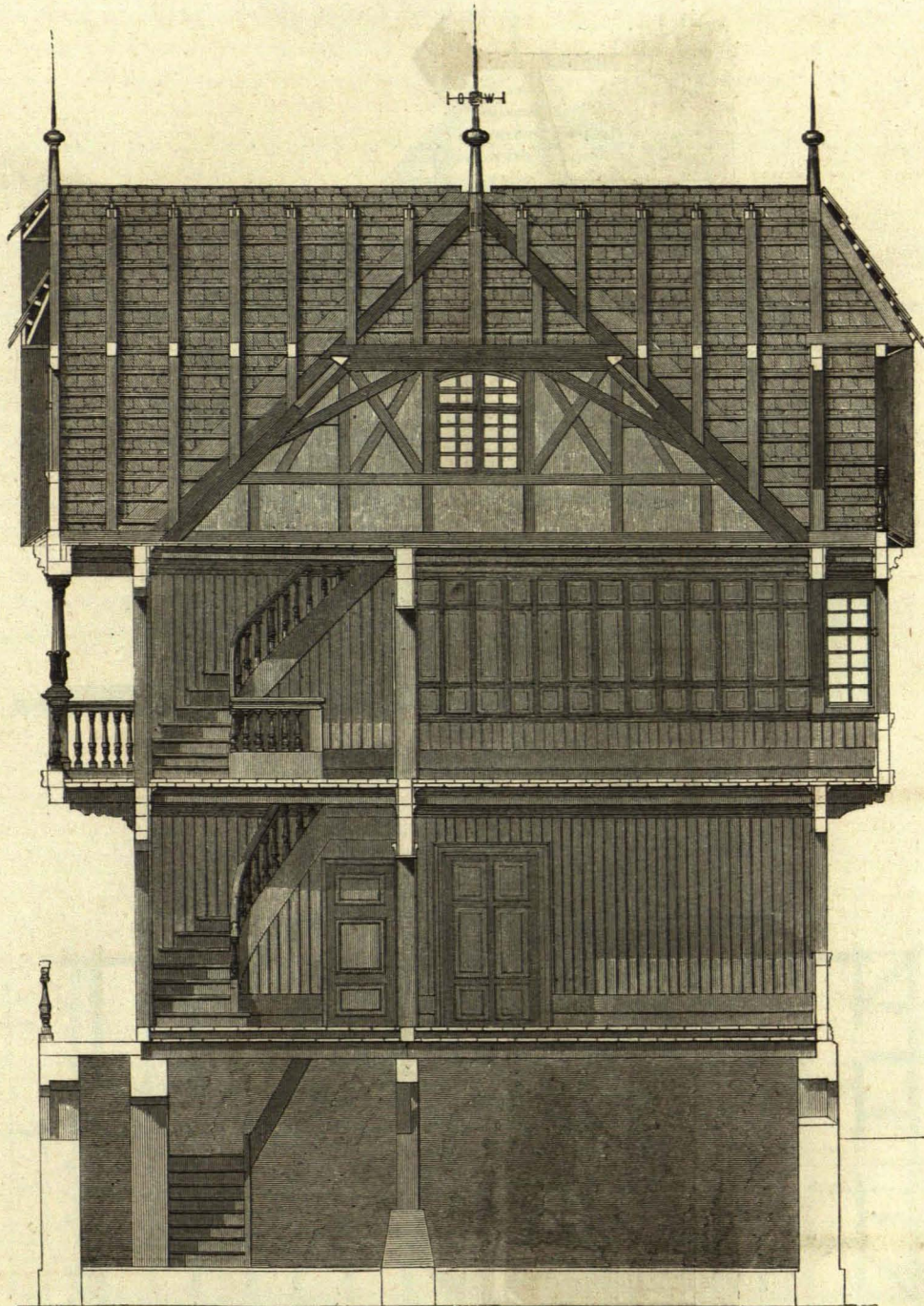
Eiläufiges Bauernhaus; Durchschnitt.
