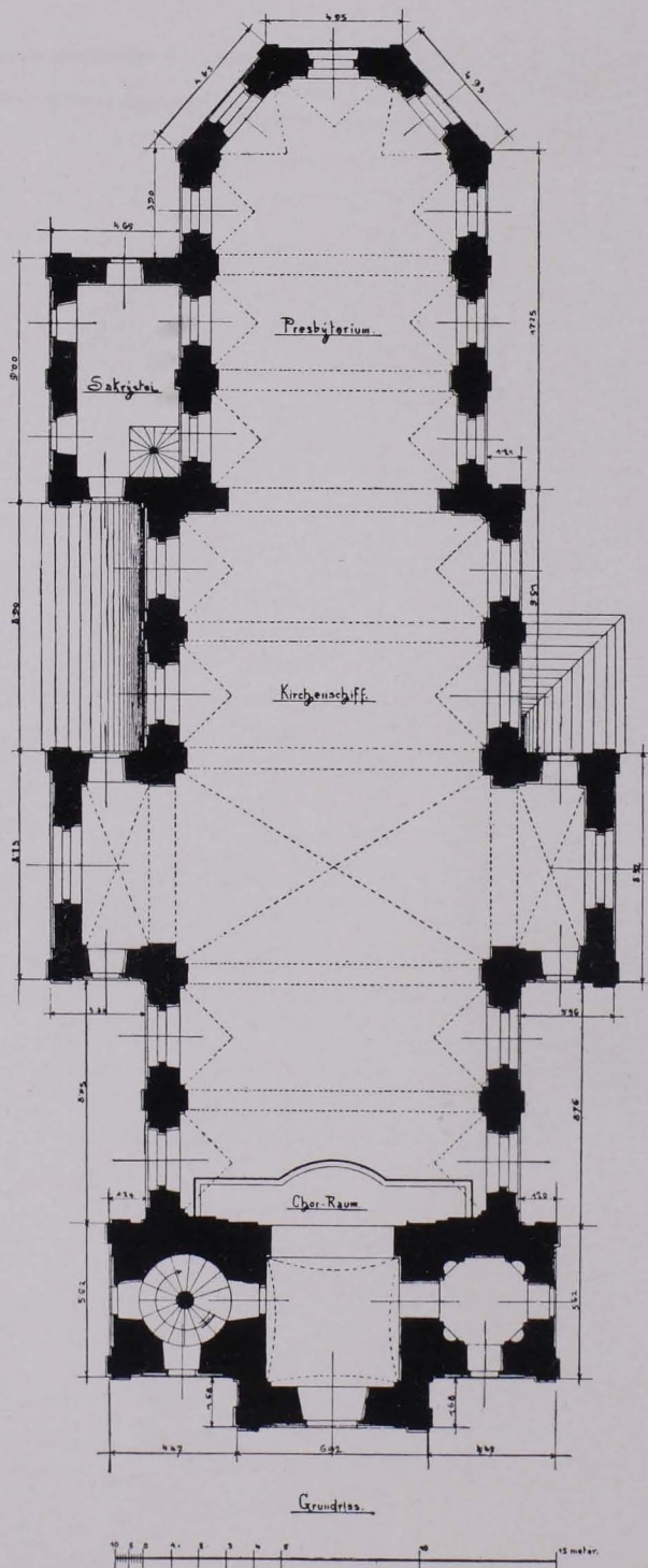
Abb. 56. Obergreogenthal. Grundriß Aufnahme der Staatsforstverwaltung Oberleutendorf, Baumeister Franz Nuska
