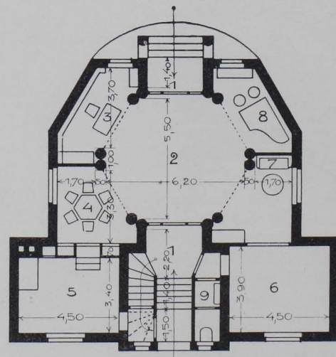
Abb. 18. Entwurf einer kleinen Sommervilla. 1904. Grundriß des Erdgeschosses
