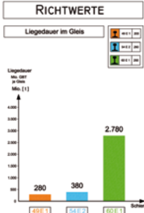
Abb. 1: Richtwerte für die Liegedauer der Schienen 49E1 (200), 54E2(260) und 60E1 (260) (Bild: Albert Jörg)
