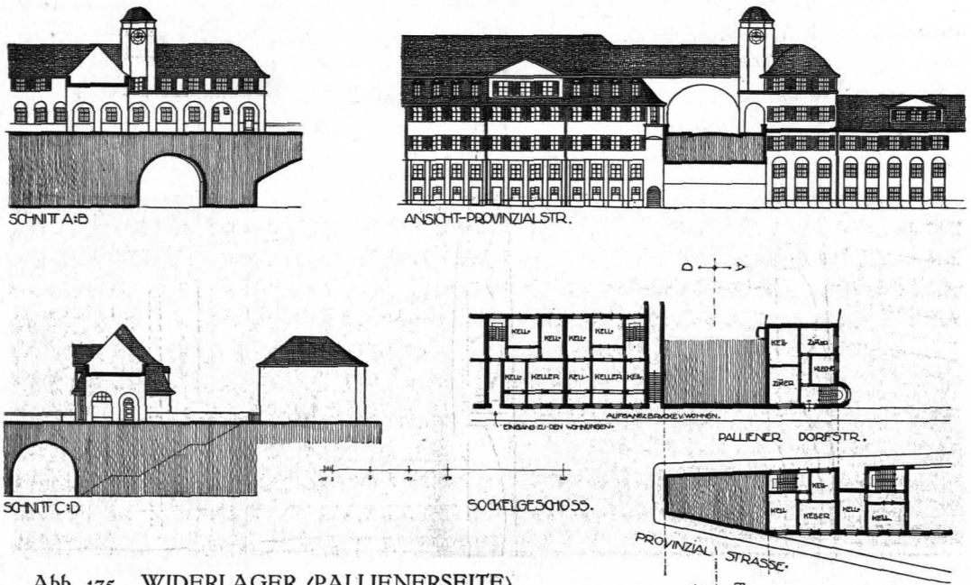
Abb. 175. WIDERLAGER (PALLIENERSEITE).
