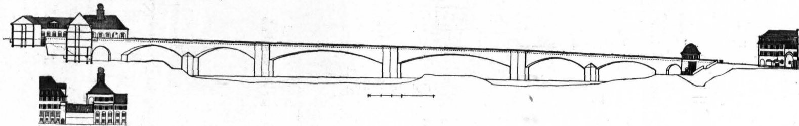
Abb. 171. ANSICHT (VARIANTE).
