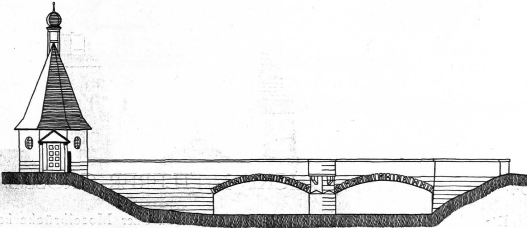
Abb. 167. HAUPTANSICHT. (M. 1:300.)
