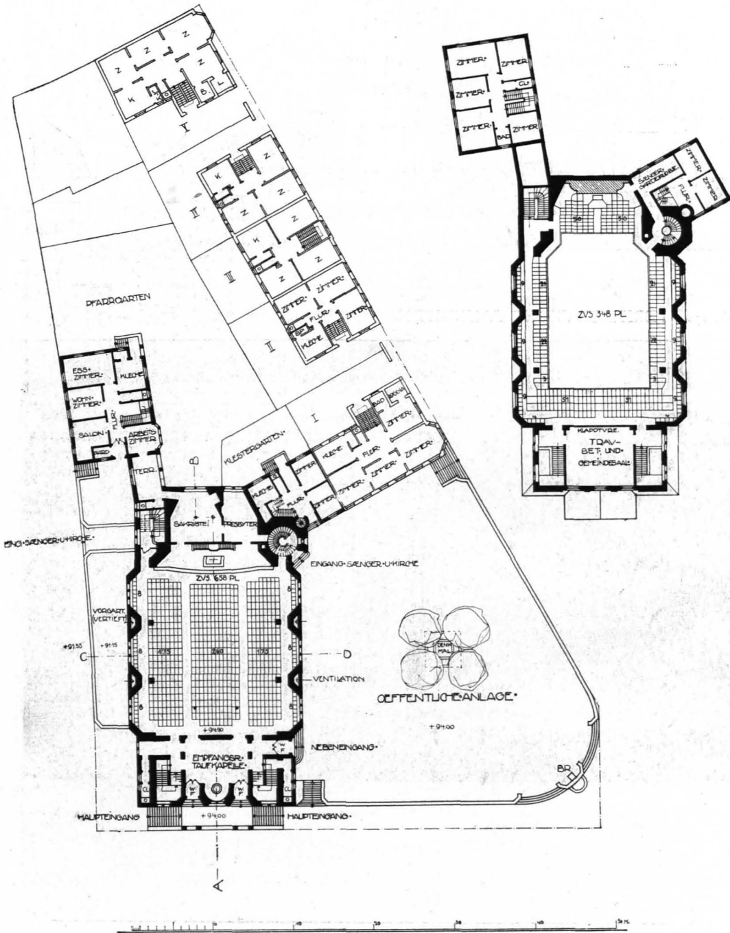
Abb. 149. GRUNDRISS DES SCHIFFES.
