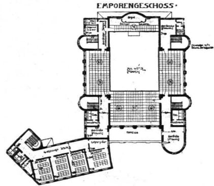
GRUNDRISS.
