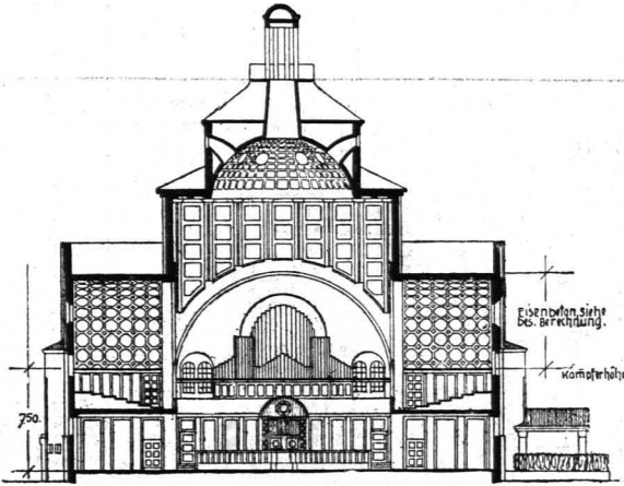
Abb. 145. SCHNITT A—B.
