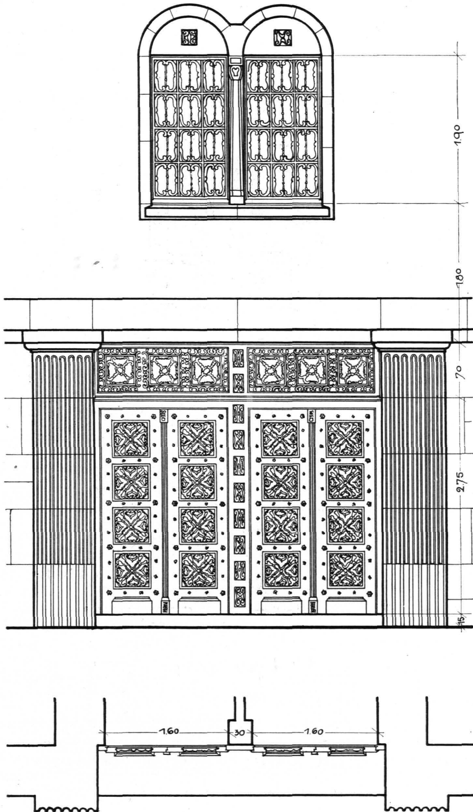
GRUNDRISS DES PORTALS.
