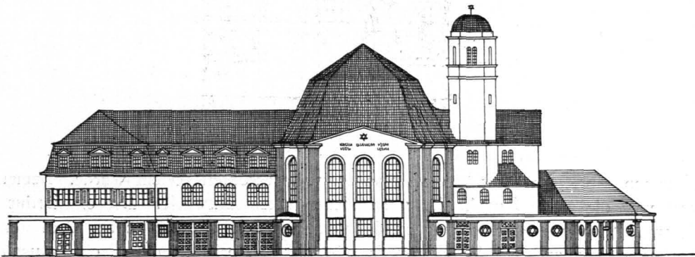
Abb. 139. ANSICHT GOETHESTRASSE.
