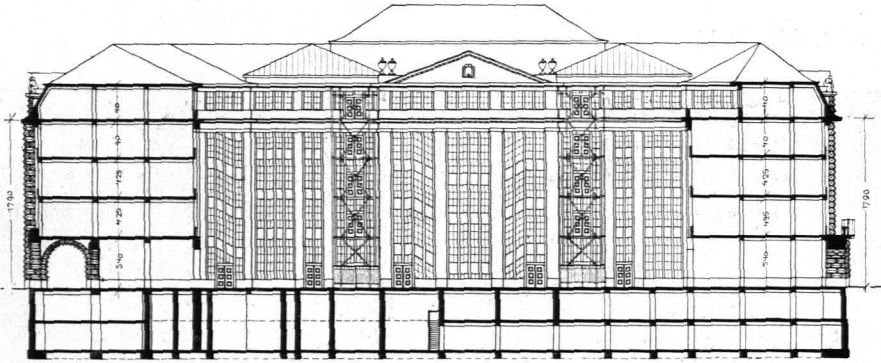
Abb. 126. SEITENANSICHT.
