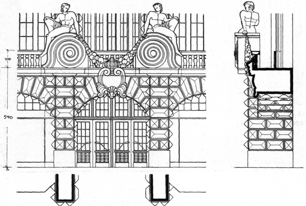
Abb. 127. PORTALDETAIL.
