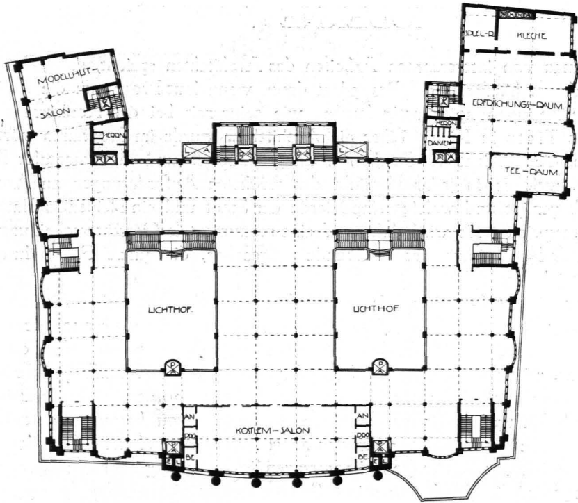
Abb. 118. I. OBERGESCHOSS.
