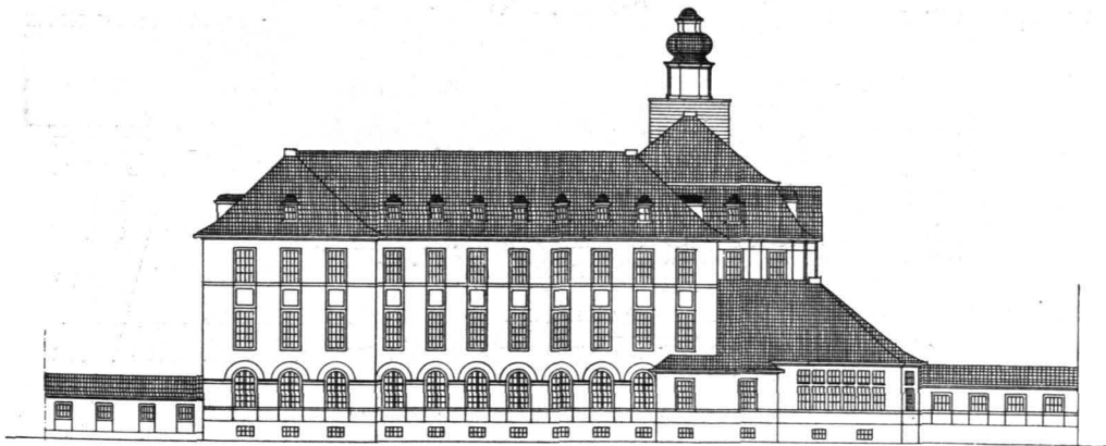
Abb. 105. ÖSTLICHE ANSICHT.
