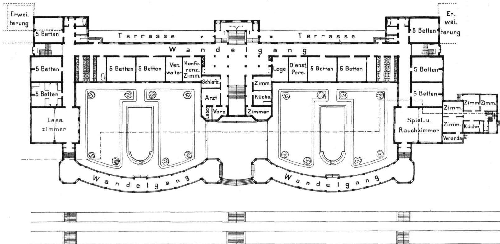
Abb. 97. DAS ERDGESCHOSS.
