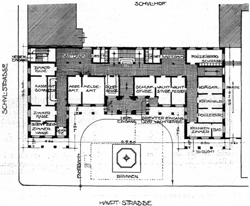
Abb. 72. ERDGESCHOSS. (M. 1:400.)
