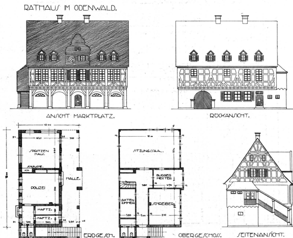
Abb. 70. ANSICHTEN UND GRUNDRISSSE. (M. 1:370.)
